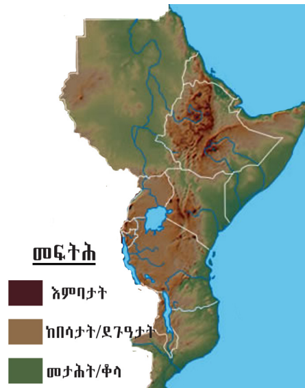
ካርታ 2.4 ቅርፂ መሬት ምብራቅ አፍሪካ
