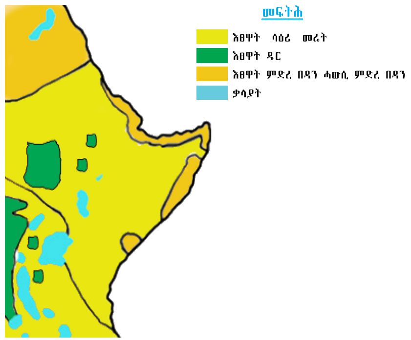
ካርታ 3.1 ዝርገሐ እፅዋት ተፈጥሮ ምብራቕ ኣፍሪካ
