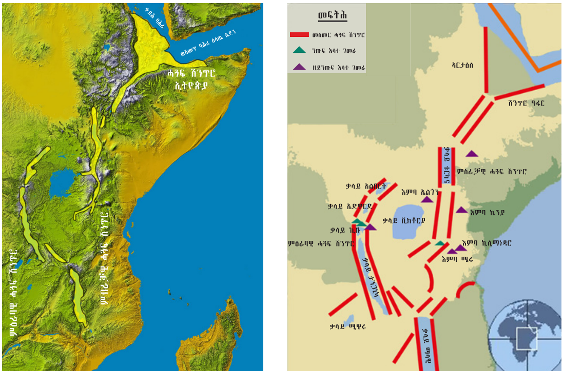
ካርታ 2.6 ዓብይ ሓንፍ ሸንጥሮ ምብራቕ ኣፍሪካ
