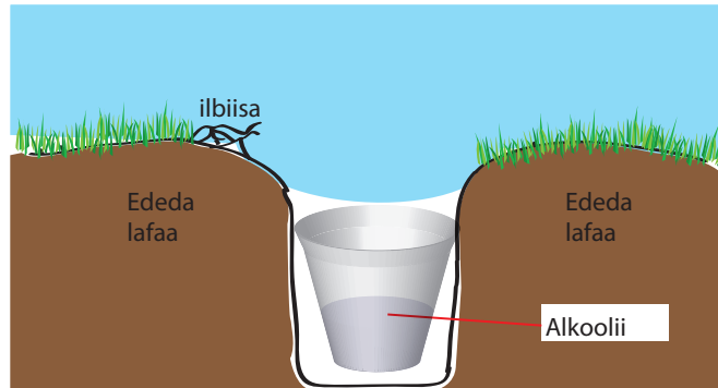
Fakkii 6.8: Kiiyessituu boollaa
