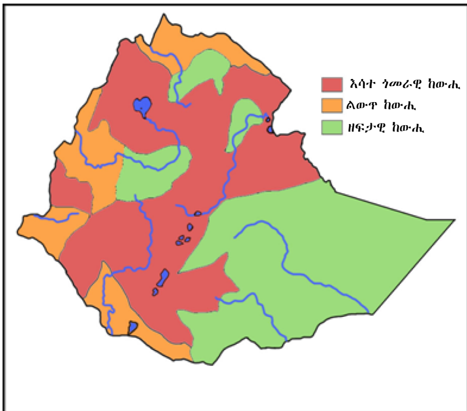
ካርታ 2.2 ዓይነታት ከውሐ ኢትዮጵያ
