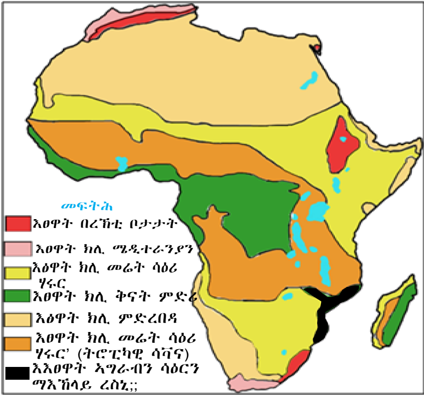
ካርታ 3.1 ዝርግሐ እፅዋት ተፈጥሮ ኣፍሪካ
