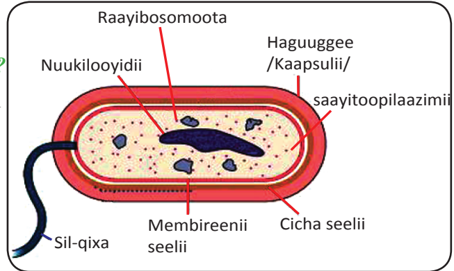
Fakkii 2.8: Seelii waliigalaa baakteeriyamii.
