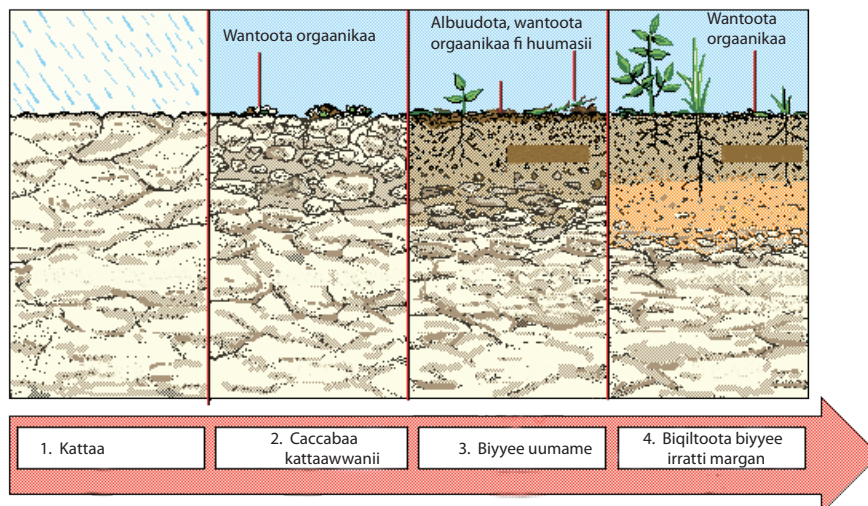
Fakkii 6.13: Adeemsa waliigalaa uumama biyyee
