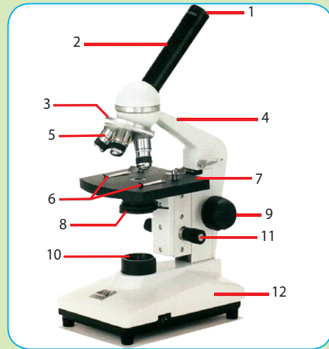
Fakkii 1.4: Qaamolee Maayikrooskooppii
